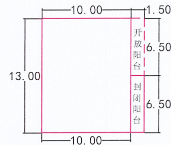
二至三层平面图 1:200
