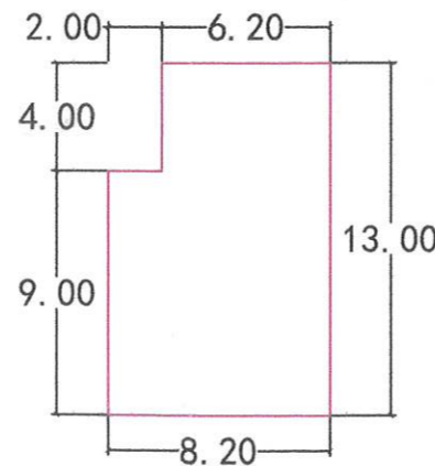
首层平面图 1:200
