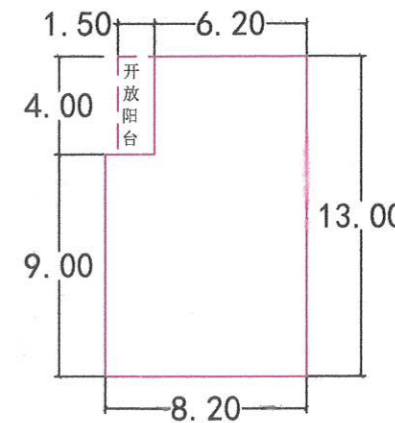
二层平面图 1:200
