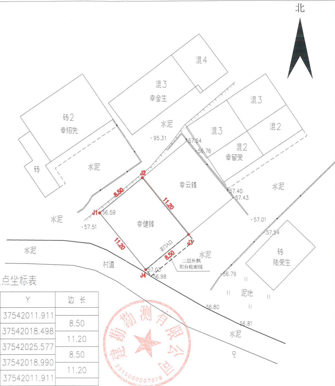
总平面图 1:300
