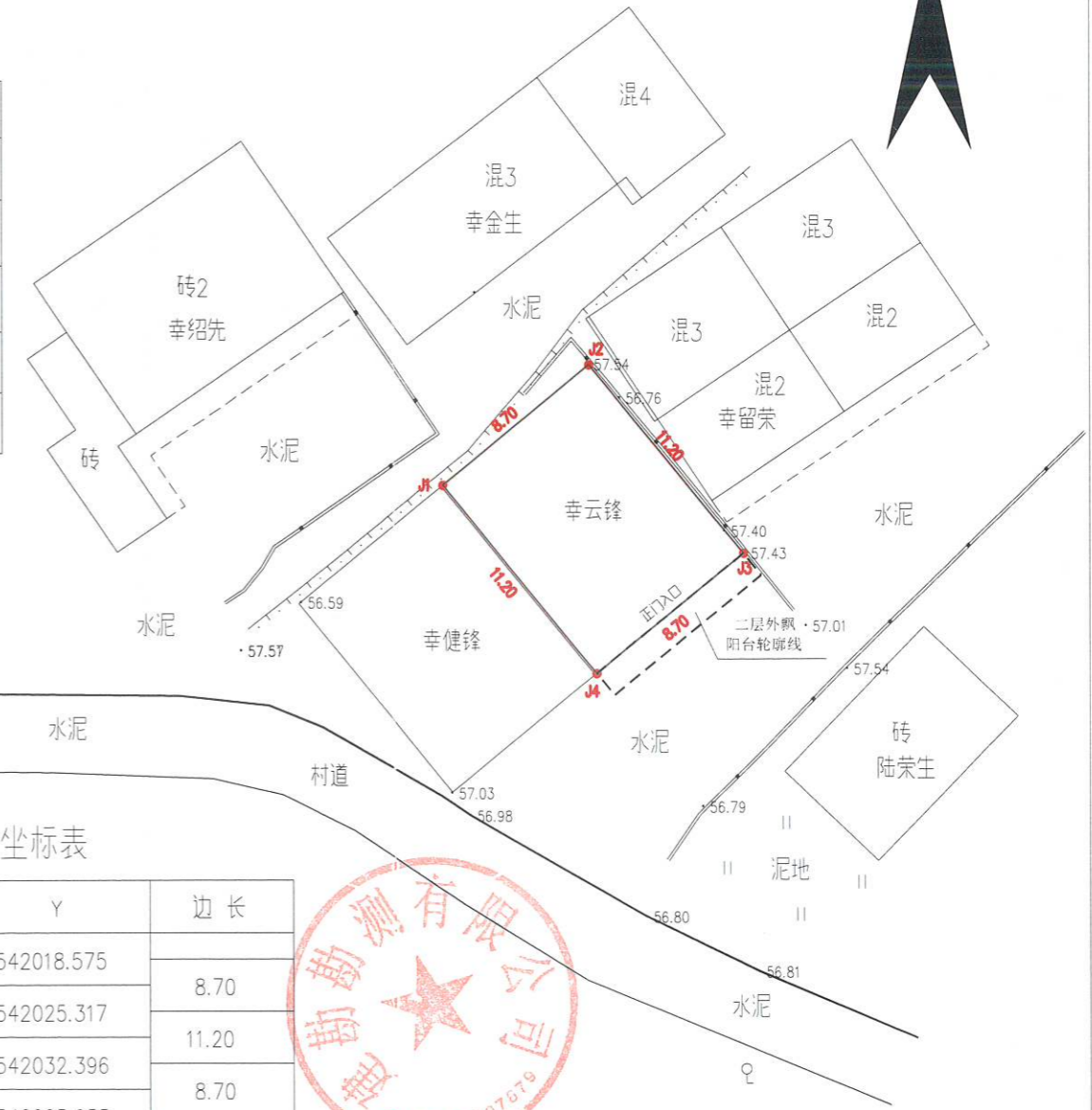
总平面图 1:300
