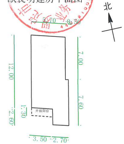
罗定市连州镇云致村委南山53号之二欧良明建房平面图
