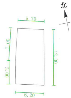
首层平面图 1:200
