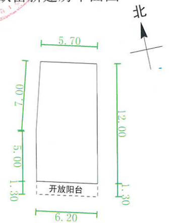
2-5层平面图 1:200
