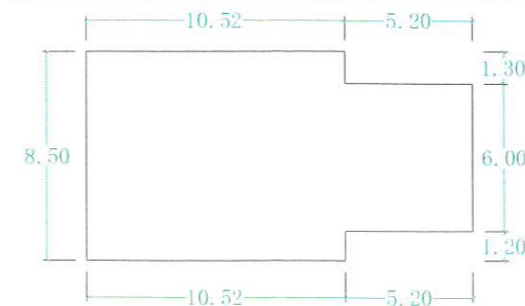
首层平面图 1:100
