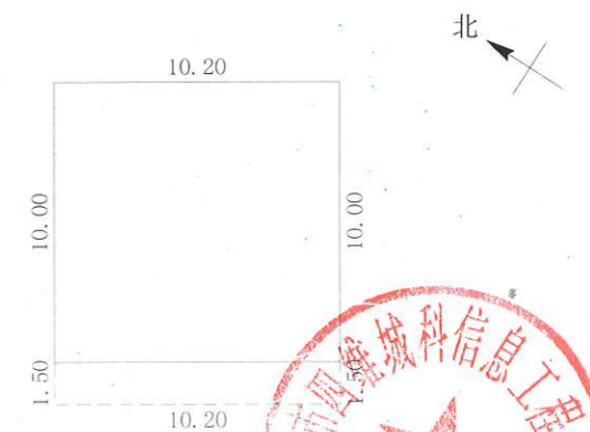
二层平面图 1:300
